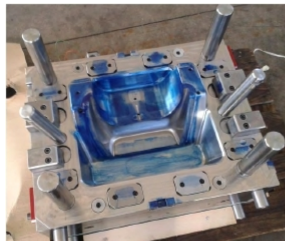
Stampo matrice "Mostrina mobiletto Fiat 520" in acciaio
